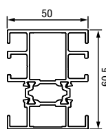
Paplašināšanas profils 50 mm
